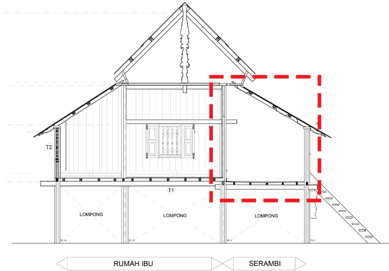
Gambar 27 Keratan ruang serambi dan rumah ibu rumah warisan Sonyum
