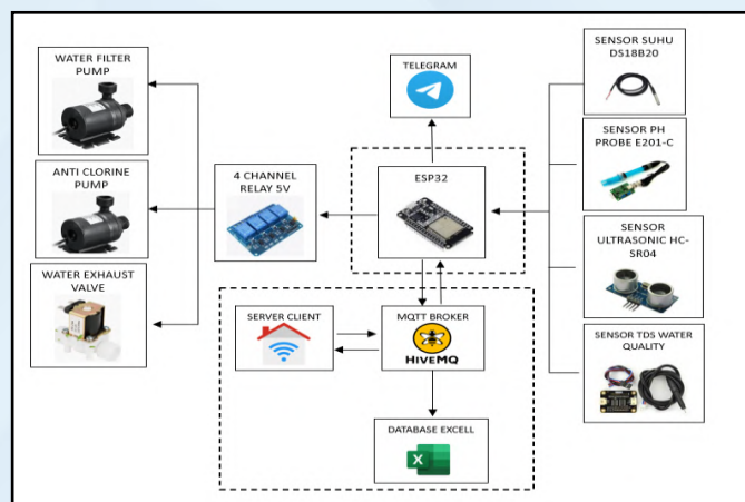
Rajah 1: Reka bentuk sistem pemantauan dan kawalan kualiti air akuaponik berasaskan IoT
