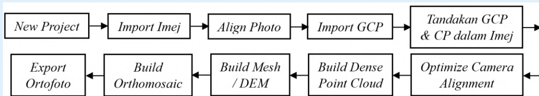
Rajah 4: Peringkat-peringkat pemprosesan menggunakan perisian Agisoft Metashape Professional untuk penghasilan ortofoto.
