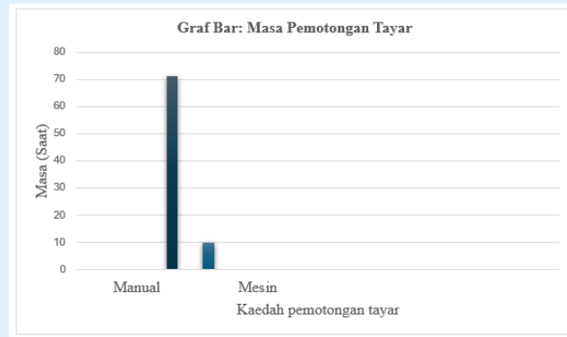
Rajah 5: Graf Bar berkenaan perbandingan masa pemotongan tayar antara kaedah manual dan automatik.
