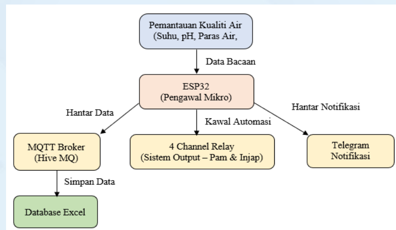
Rajah 2: Aliran proses sistem pemantauan dan kawalan kualiti air akuaponik berasaskan IoT
