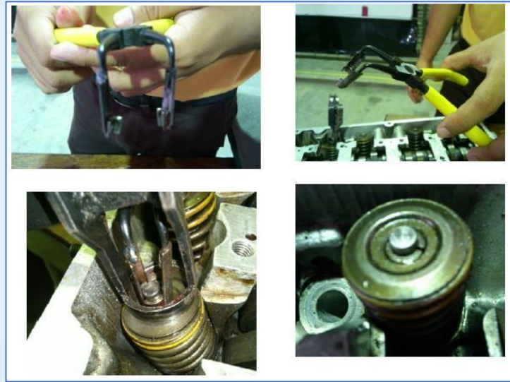
Rajah 2: Kaedah pemasangan valve keepers menggunakan alat inovasi
