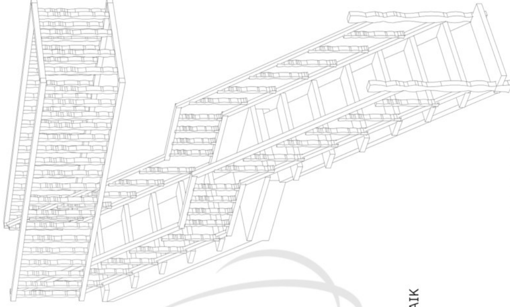
PANDANGAN ISO
