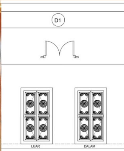
1940 MM X 1100 MM 2 BUKAAN PINTU KAYU YANG BERCORAK BUNGA DIPERBUAT DARIPADA KAYU CENGAL BESERTA UKIRAN MENGIKUT PERINCIAN
