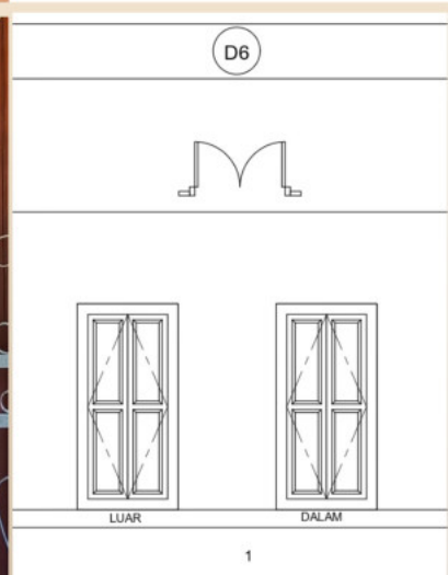
1940 MM X 950 MM 2 BUKAAN PINTU PANEL DENGAN BINGKAI KAYU ( KAYU CENGAL ) BESERTA UKIRAN MENGIKUT PERINCIAN
