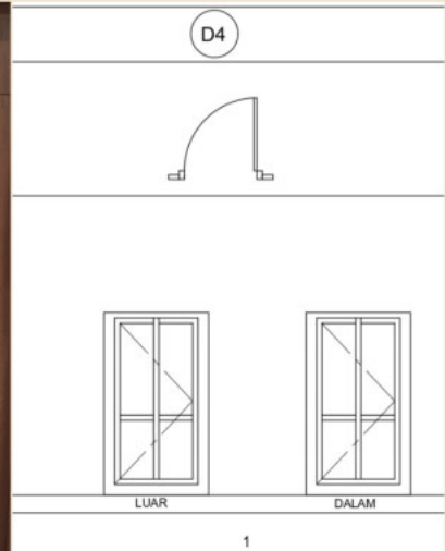
1710 MM X 780 MM 2 BUKAAN PINTU PANEL DENGAN BINGKAI KAYU ( KAYU CENGAL ) BESERTA UKIRAN MENGIKUT PERINCIAN
