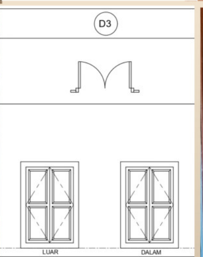
1650 MM X 1110 MM 2 BUKAAN PINTU PANEL DENGAN BINGKAI KAYU ( KAYU CENGAL ) BESERTA UKIRAN MENGIKUT PERINCIAN
