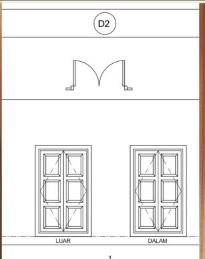
1830 MM X 1130 MM 2 BUKAAN PINTU PANEL DENGAN BINGKAI KAYU ( KAYU CENGAL ) BESERTA UKIRAN MENGIKUT PERINCIAN
