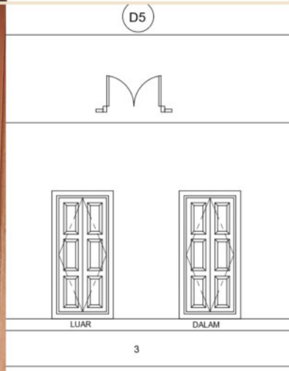
1830 MM X 880 MM PINTU PANEL KAYU ( KAYU CENGAL ) BESERTA UKIRAN MENGIKUT PERINCIAN
