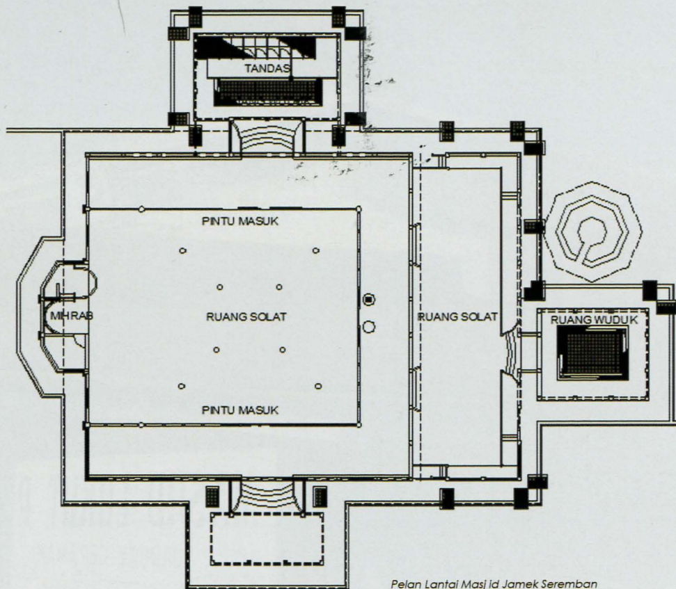
Pelan Lantai Masjid Jamek Seremban
