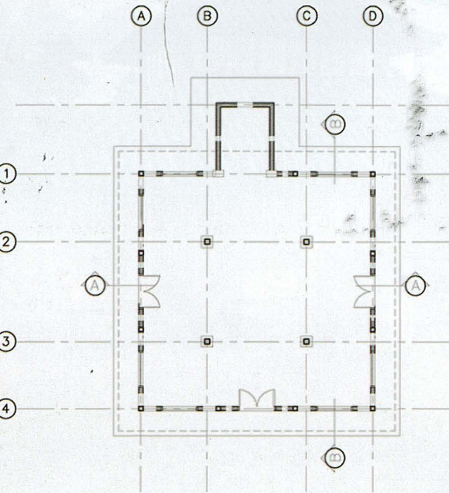
Pelan Lantai Masjid
