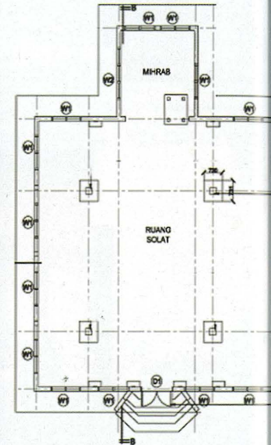
Pelan lantai Masjid Kariah Tanah Air Hitam
