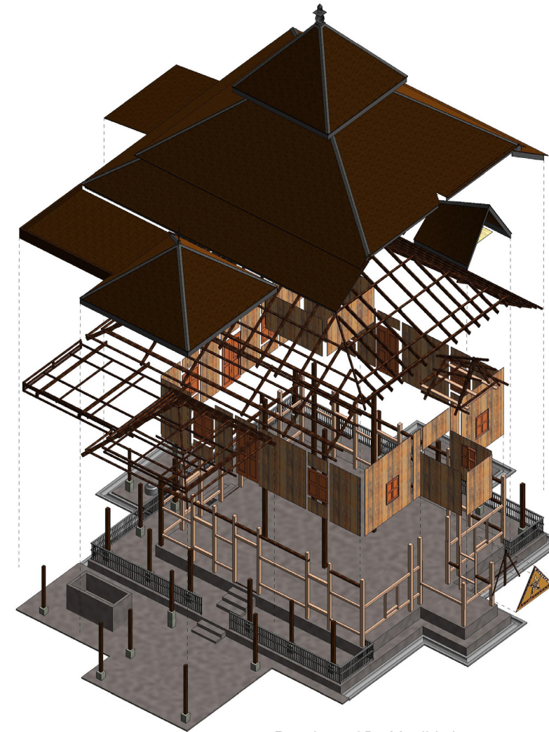
Pecahan 3D Masjid Lama Kampung Tanjung Beringin
