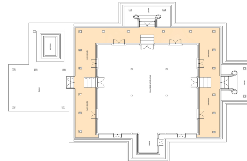
Ruang serambi yang berada pada bahagian hadapan, belakang dan kiri masjid
