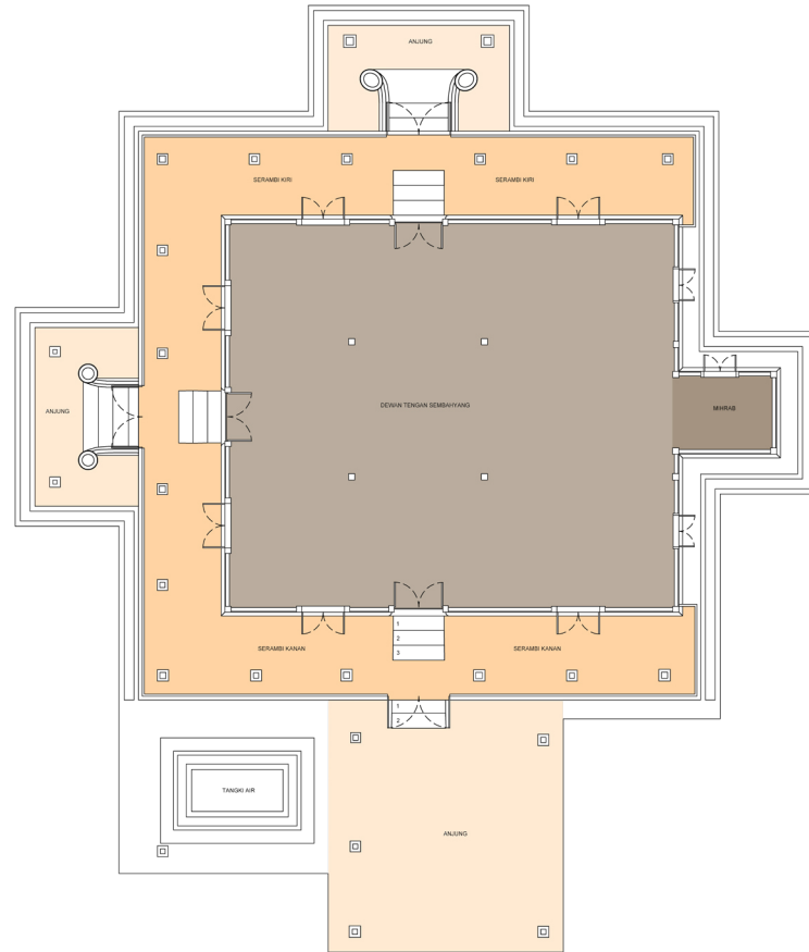
Pelan Lantai Masjid Lama Kampung Tanjung Beringin
